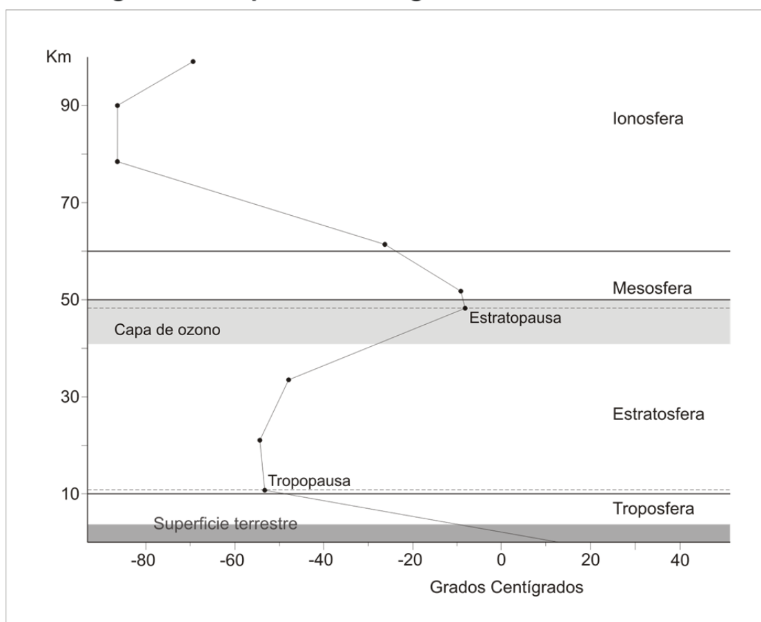
Figura 1 - Esquema estratigráfico de la atmósfera
